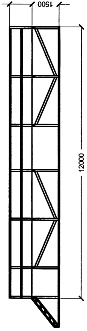
Bühnenlängsschnitt M=1:100
