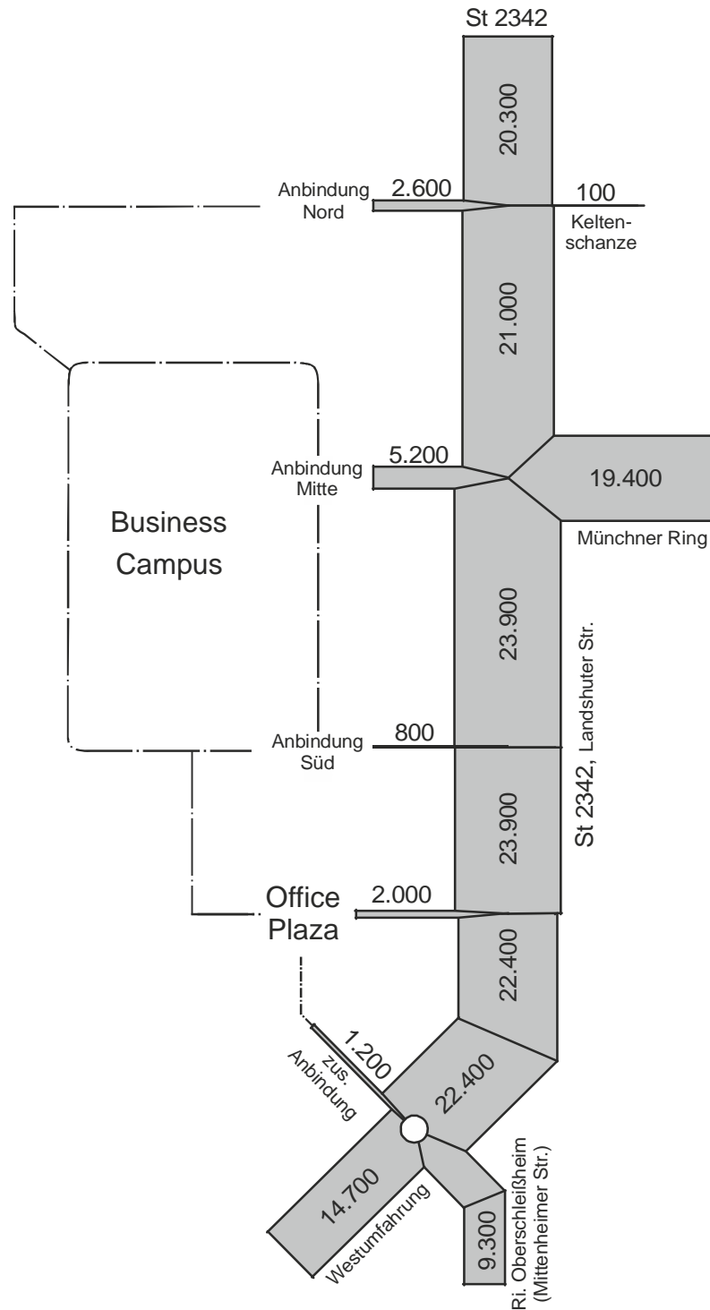
Abb. 4: Querschnittsbelastungen St 2342 im Bereich Business Campus Gesamtverkehr in Kfz/24 Stunden Prognose 2030 mit Business Campus, Office Plaza und Westumfahrung Oberschleißheim Variante mit zusätzlicher Anbindung Office Plaza an die Westumfahrung
